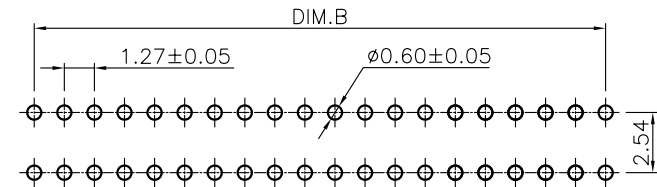
P.C.B. LAYOUT
